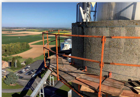
Echafaudage en Consoles en cours de montage sur cheminée de 80m
